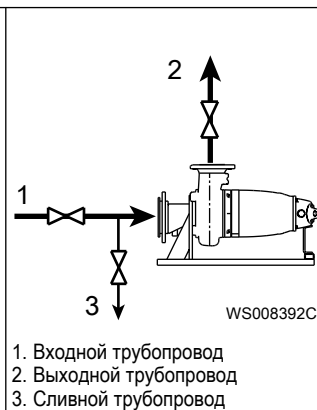
Рис. 23: Вариант Z (показан типовой насос)
