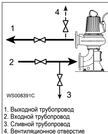
Рис. 22: Вариант Т (показан типовой насос)
